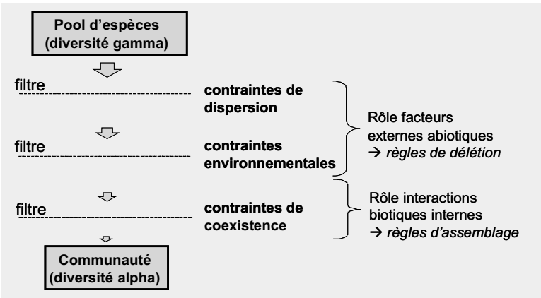
FIGURE 2 : Règles d'assemblage et règles de délétion dans les communautés végétales (d'après KEDDY, 1992).
