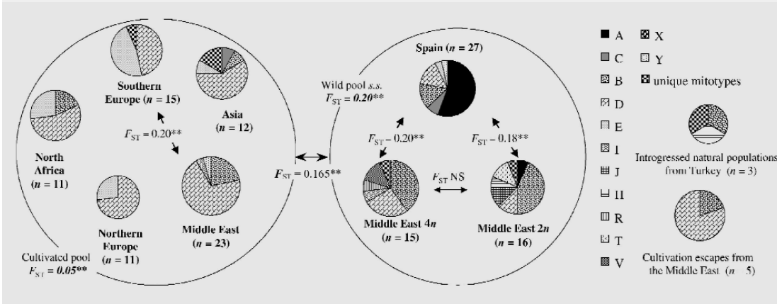
FIGURE 3 : Composition des deux pools (cultivé et sauvage) de Medicago sativa ( sensu lato ) et niveaux de différenciation entre les différents groupes. Seules les valeurs significatives des F_{st} sont indiquées. Les différents motifs représentent la proportion des différents cytotypes au sein des groupes (d'après MULLER et al. , 2003).
