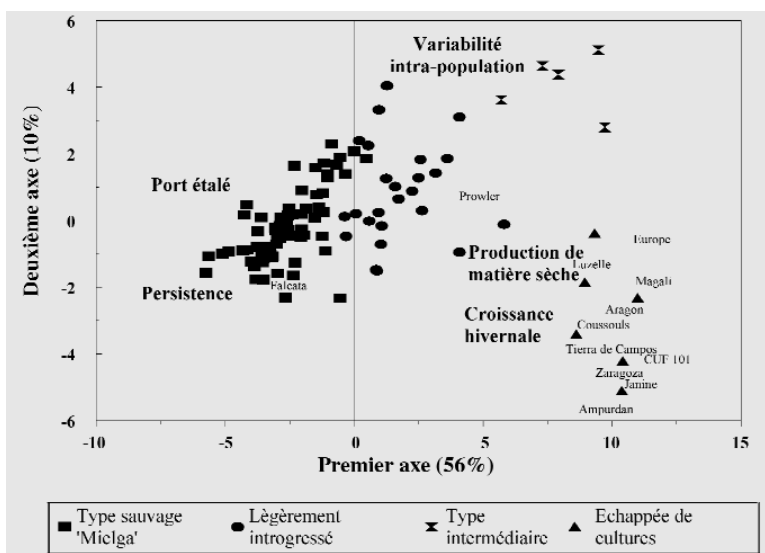
FIGURE 2 : Représentation des deux premiers axes de l'analyse en composantes principales réalisée sur les données agronomiques et position des 102 populations naturelles de Medicago sativa collectées en Espagne, de 12 cultivars et d'un écotype de Medicago sativa subsp. falcata .
