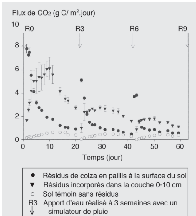
FIGURE 2 : Effets de la localisation de résidus de colza dans une colonne de sol (en laboratoire) sur les flux de CO 2 émis au cours de la décomposition.
