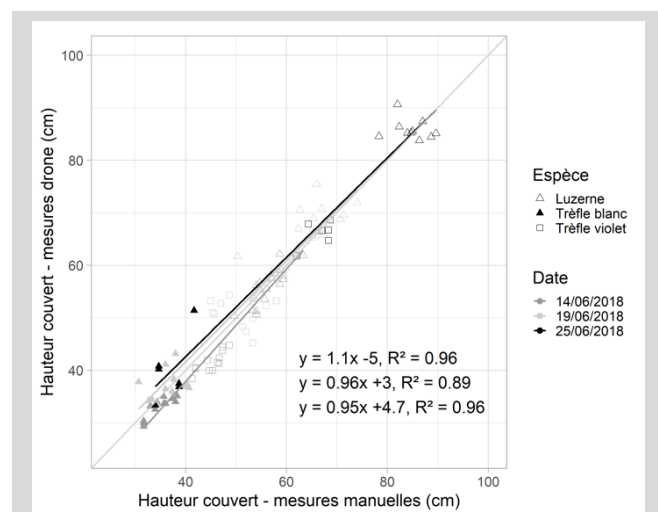
FIGURE 1 : Relation entre les hauteurs mesurées à la règle et celles estimées par photogrammétrie pour les légumineuses le 14/06, 19/06 et 25/06.
