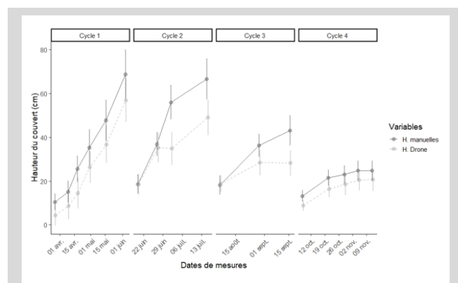
FIGURE 2 : Hauteurs moyennes (cm) des couverts de luzerne mesurées manuellement et par photogrammétrie au cours des 4 cycles de repousse sur l'essai 2.
