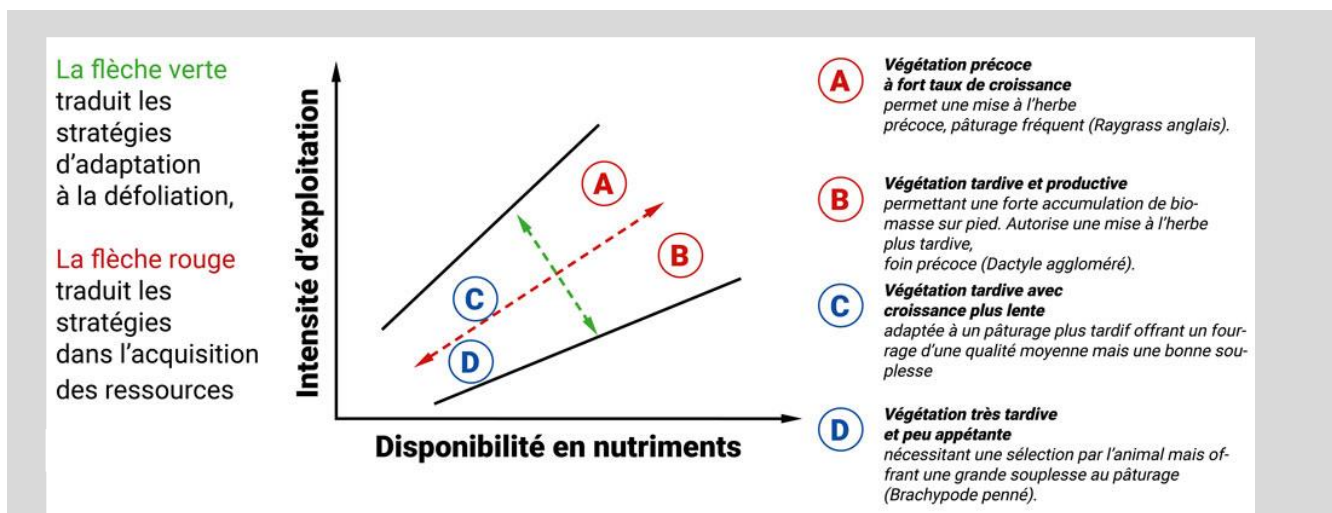
FIGURE 1 : Réponses fonctionnelles de quelques espèces de graminées en fonction de la disponibilité en nutriment du milieu et de l'intensité d'exploitation (Source : exposition Innov'herbe, 2020 https://innovherbe.bu.uca.fr/prairies-diversite/ecologie-fonctionnelle ; librement adapté de Cruz et al. , 2002)
