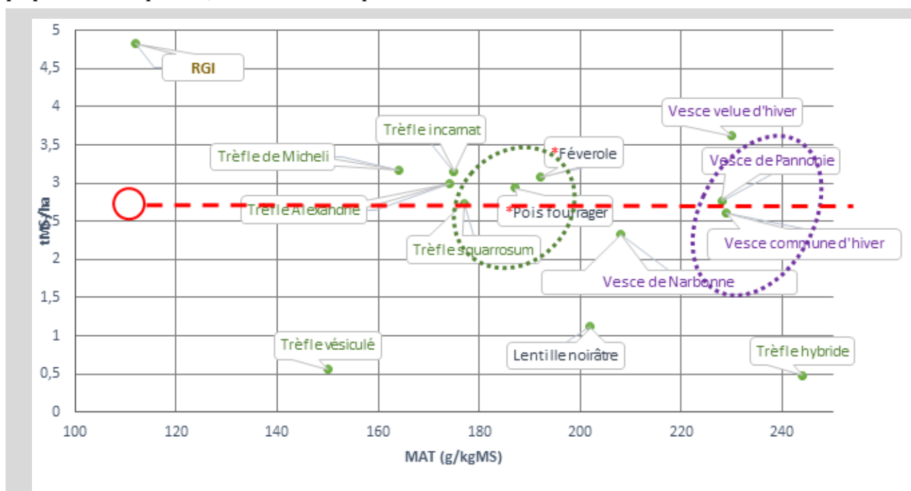
FIGURE 3 : Graphique représentant le rendement (tMS/ha) en fonction de la teneur en MAT (g/kg de MS) pour chaque espèce en première coupe. (données ajustées selon le site). *L'implantation du pois fourrager et de la féverole ne correspond pas à la date optimale pour ces espèces Figure 3 : Graph showing yield (tMS/ha) as a function of MAT content (g/kg DM) for each first-cut species. (data adjusted according to site). *Field pea and faba bean planting dates are not optimal for these species.
